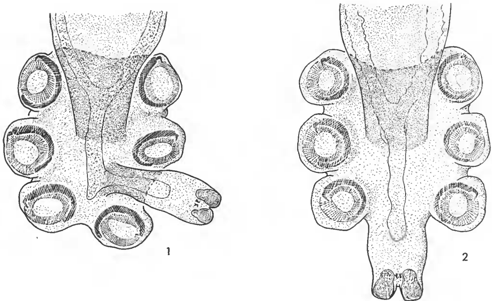
FIG. 1. — Morphologie du hapter chez Epicotyle n. g. FIG. 2. — Morphologie du hapter chez Erpocotyle Van Beneden et Hesse, 1863.
